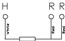
3-tråds koppling
