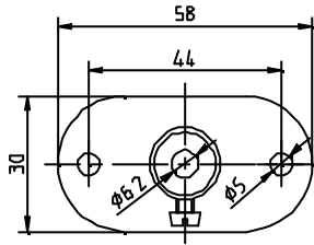
Konsol BR6.2
